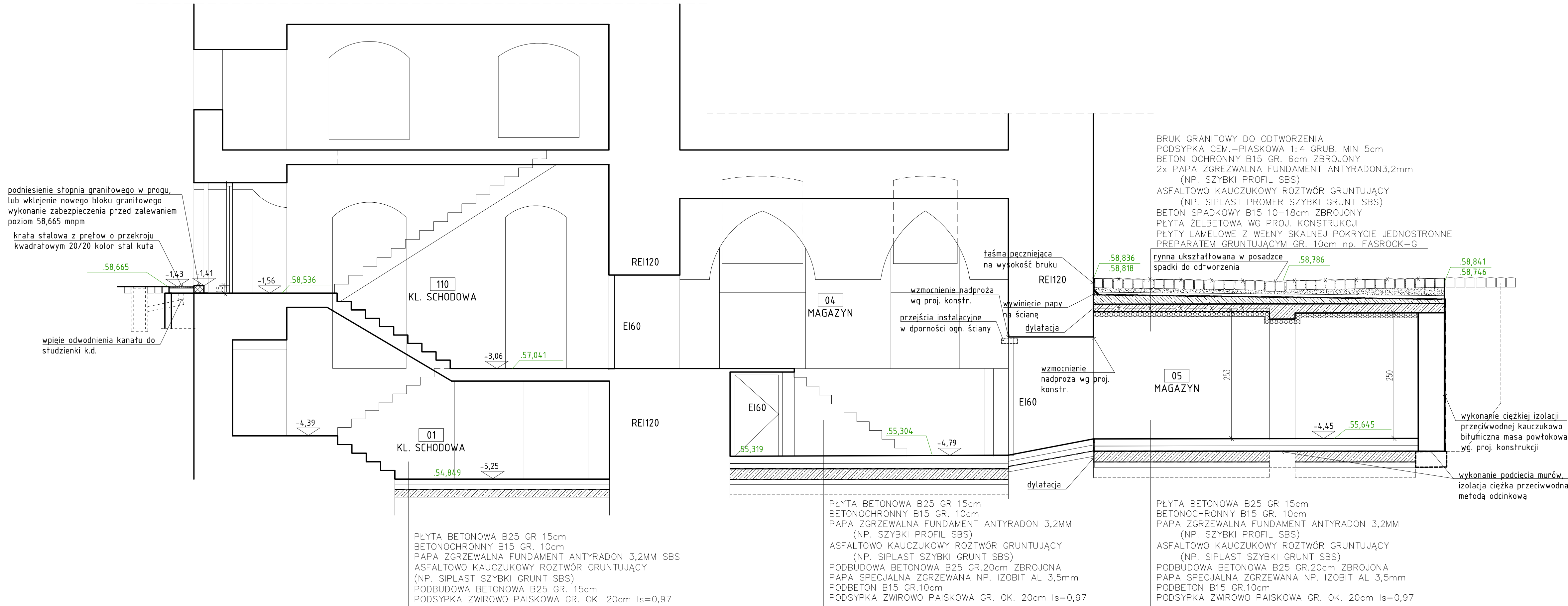
PRZEKRÓJ B-B
