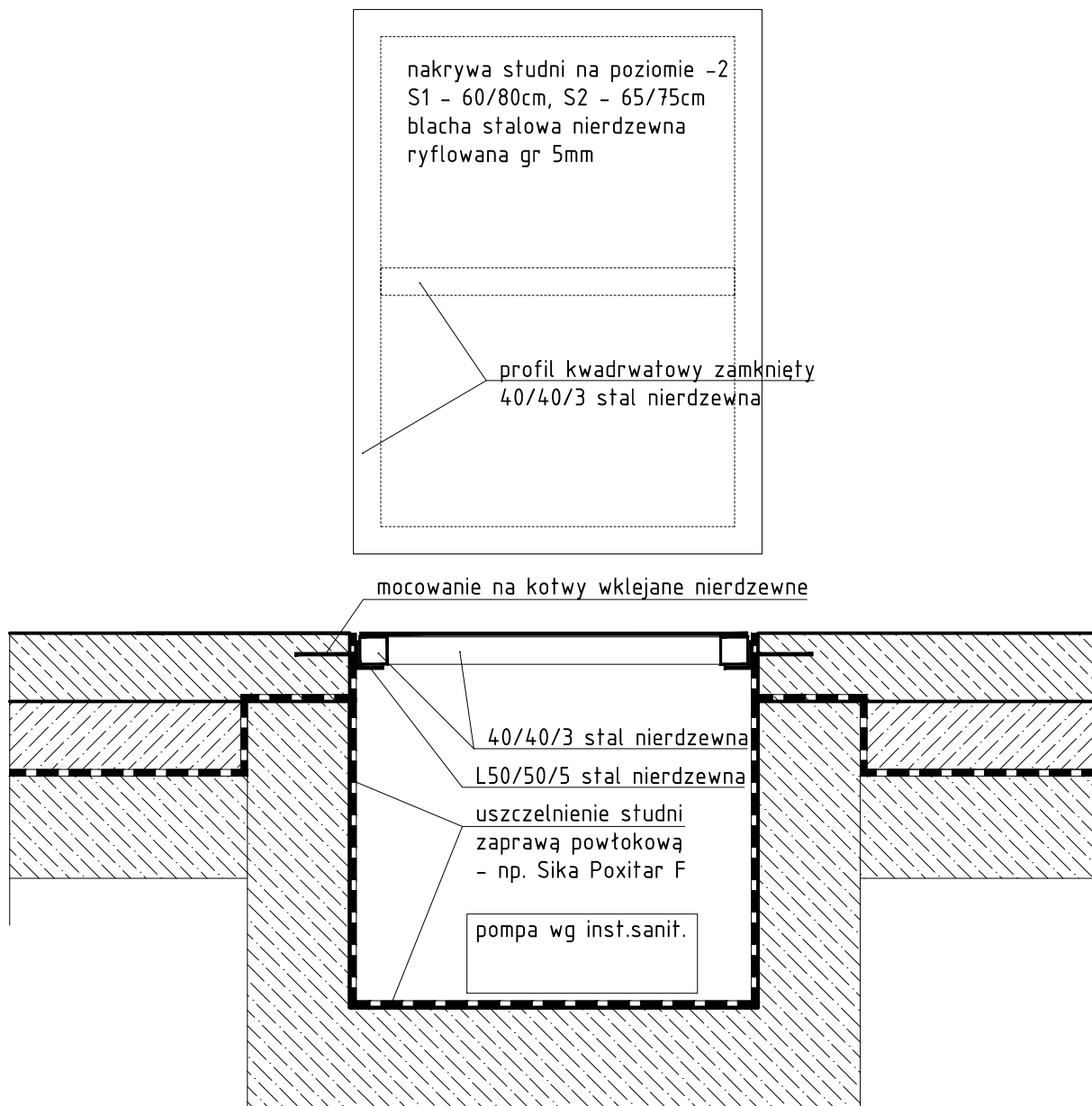
POKRYWA STUDNI [poziom -2]
