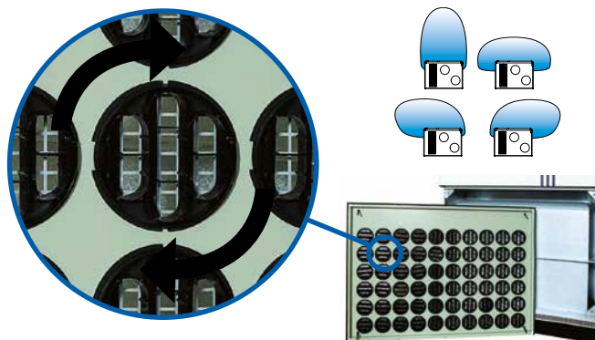
Dysze VARIZON
